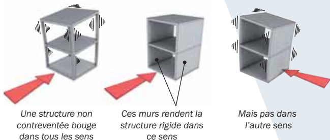
Rôle des murs de contreventement
