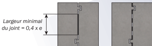
Exemples de joints verticaux collés
