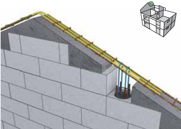
Détail d'une jonction en tête de pignon
