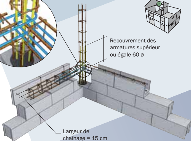
Détail d'une jonction d'angle en L
