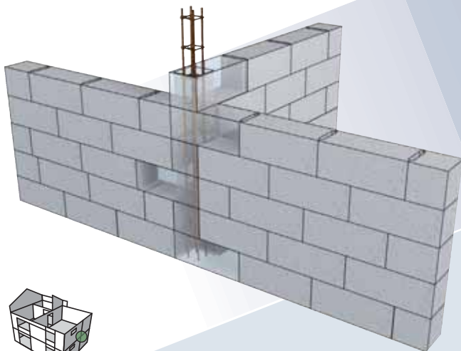
Jonction par harpage entre mur de façade et mur de refend (recommandée pour les locaux non chauffés, par exemple sous-sol)
