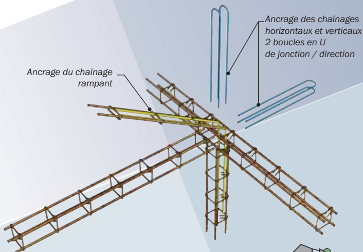
Détail d'une jonction d'angle en T avec le chaînage du rampant
