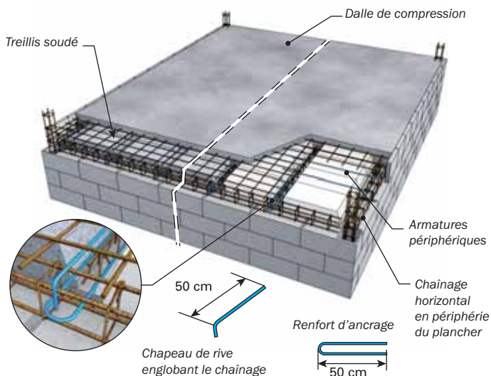
Détails des chaînages aux jonctions entre murs et planchers
