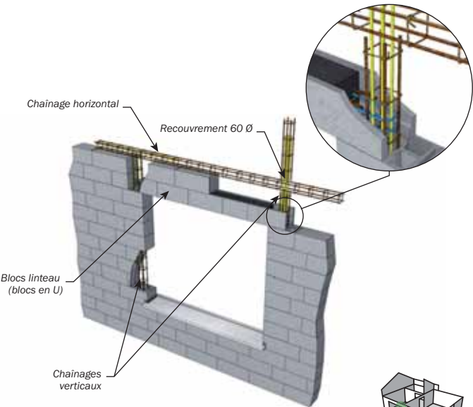
Détails des jonctions autour d'une ouverture
