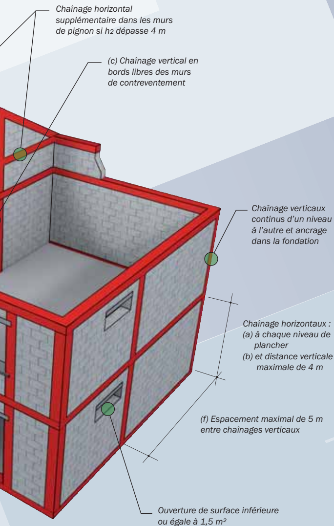
Emplacement des chaînages pour les constructions parasismiques
