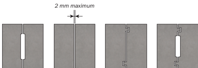
Exemples de joints verticaux non remplis
