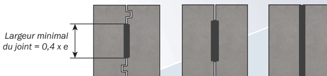
Exemples de joints verticaux maçonnés
