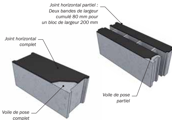
Joint horizontal épais complet (à gauche) ou partiel (à droite)
