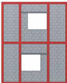
Traitement des ouvertures décalées*
